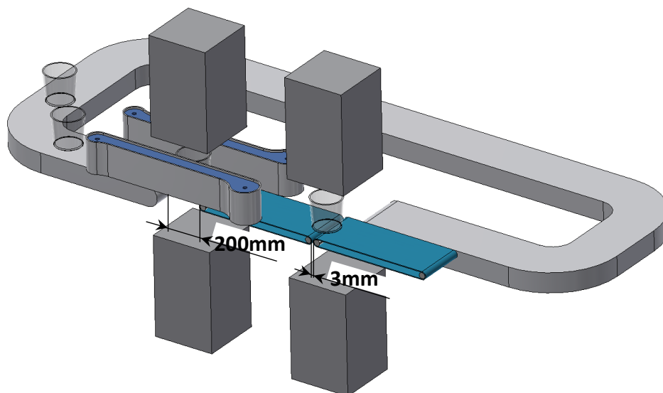
Rys.1 Widok ogólny struktury zestawu transporterów
